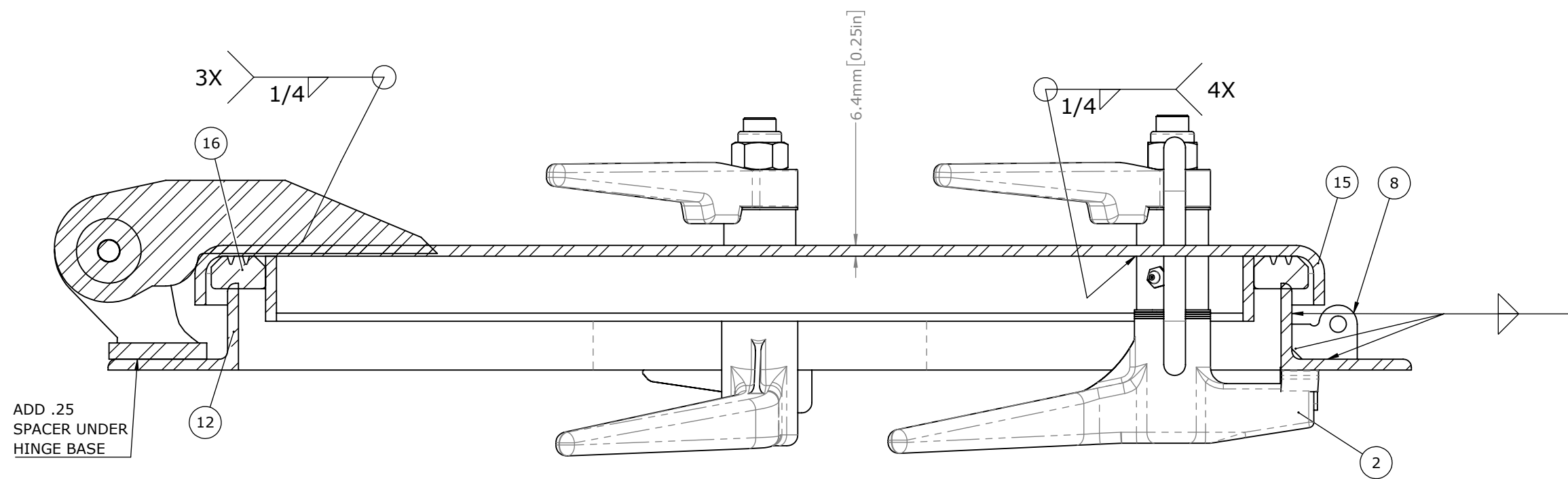
SECTION B-B SCALE 1 : 3
