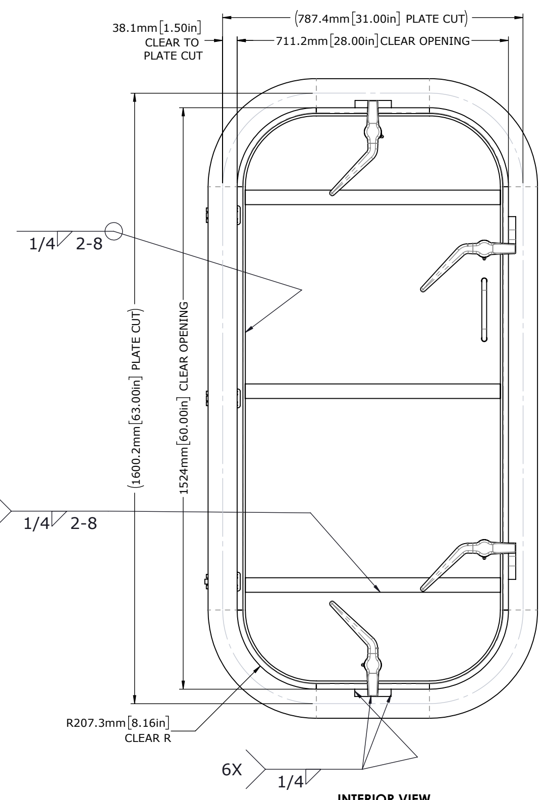
SECTION A-A
