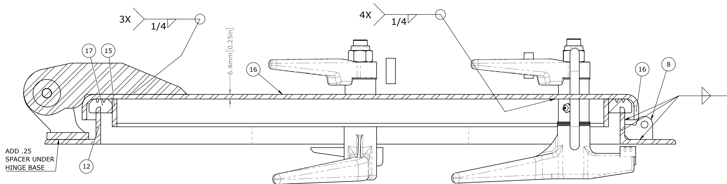
SECTION B-B SCALE 1 : 3
