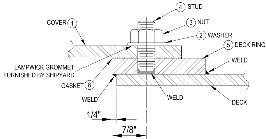
STUD DETAIL
