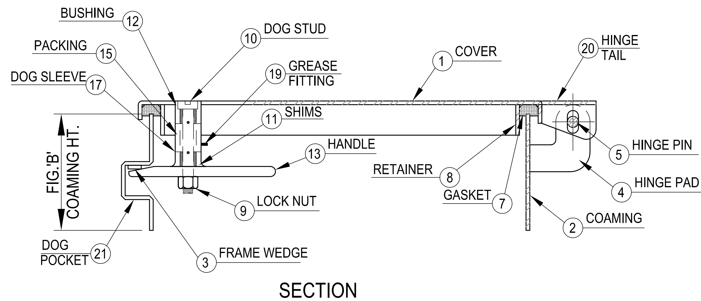
SECTION 'B-B'
