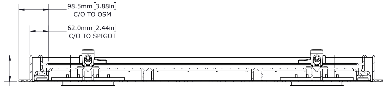
SECTION A-A SCALE 1 : 6
